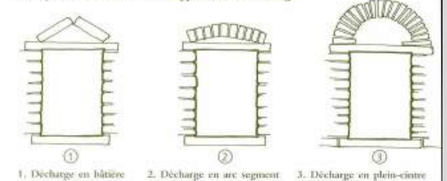
Exemples de cadres de baies non appareillés, avec décharges
