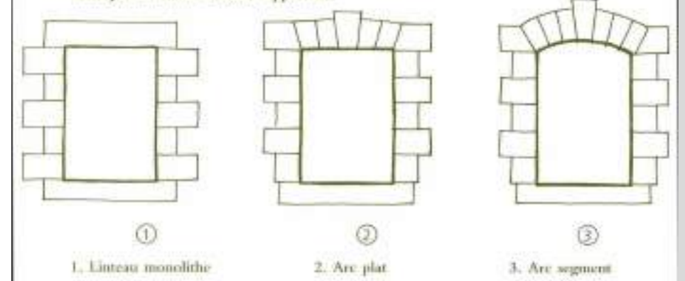
Exemples de cadres de baies appareillés
