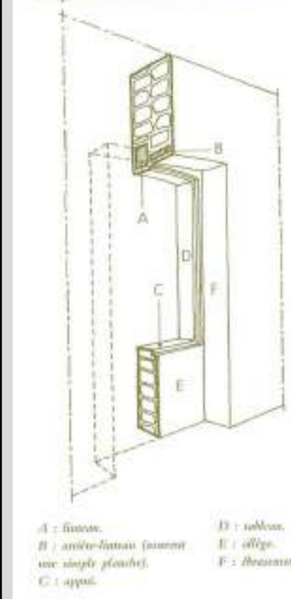
Coupe d'une baie d'un mur ordinaire
